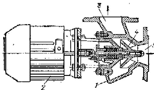
Рис. II.66. Диагональный насос ЦНПС 1 — разъемный чугунный корпус; 2 — фланцевый электродвигатель; 3 — нагнетательный патрубок; 4 — рабочее колесо; 5 — всасывающий патрубок
