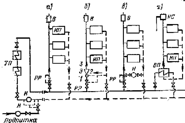
Рис. 11.24. Схемы присоединения систем отопления к водяной тепловой сети
