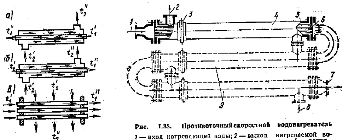
Рис. 1.37. Схемы теплообменников
