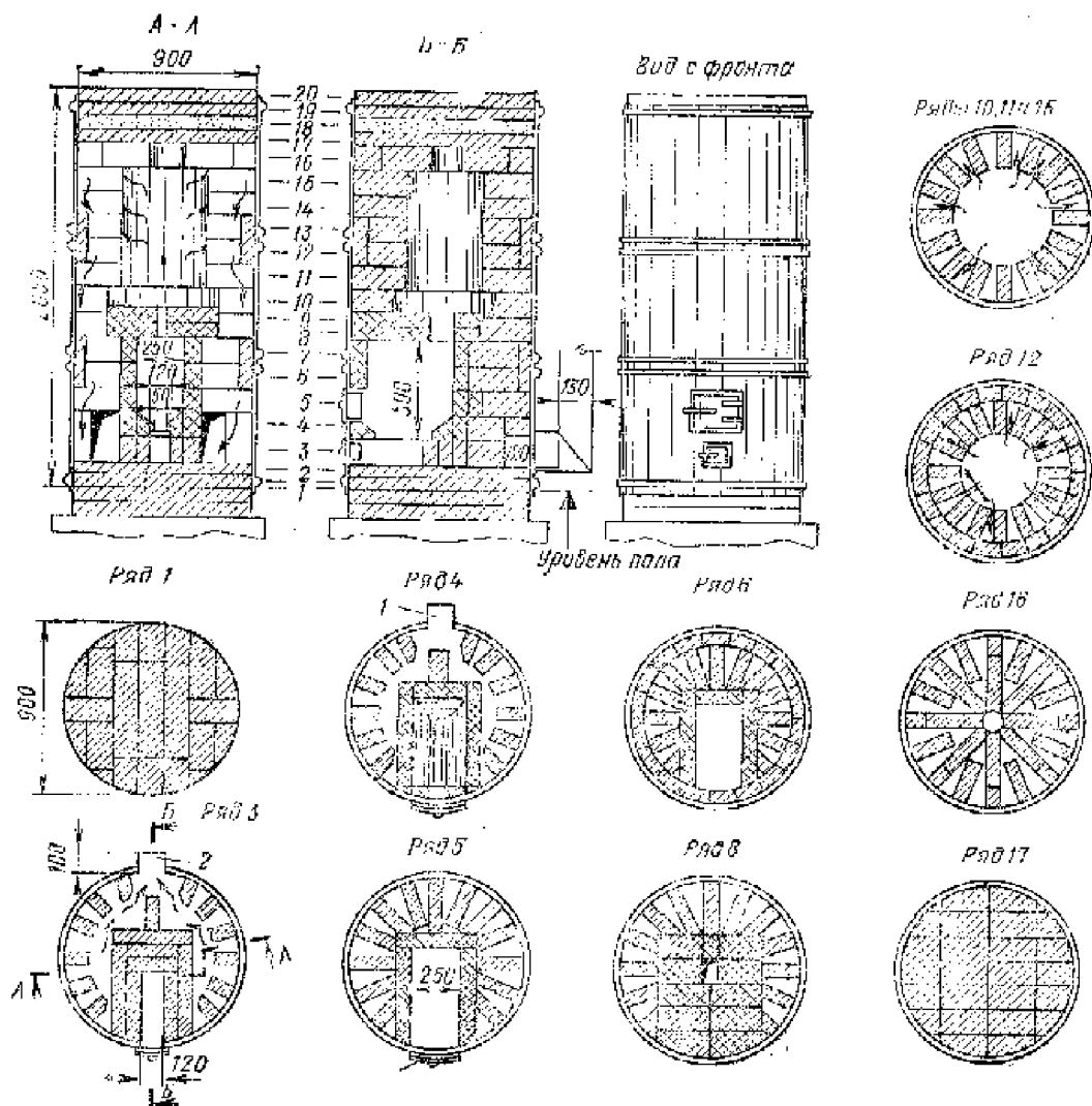
Рис. 11.91. Печь «Геркулес» 1 — патрубок d=125 ; 2 — выход дыма
