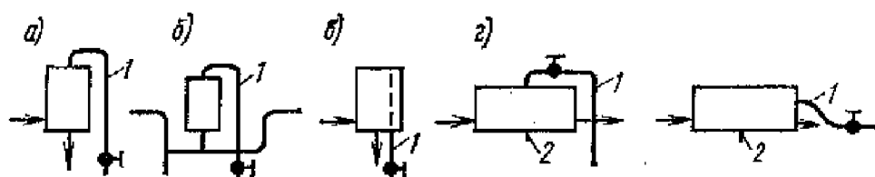
Рис. II.63. Воздухоотборники
