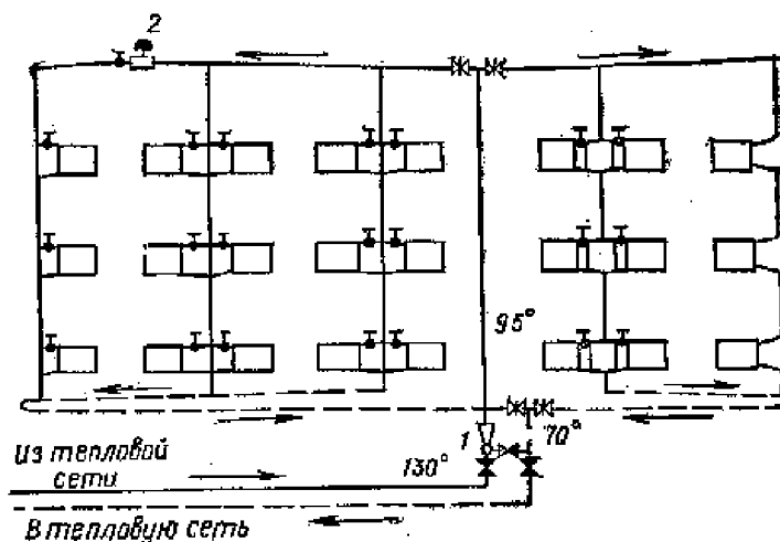
Рис. II.68. Элеватор
