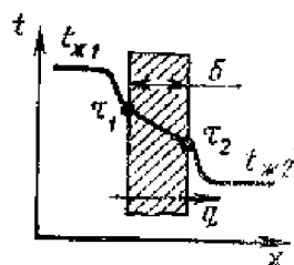
Рис. 1.35. Теплопередача через плоскую стенку
