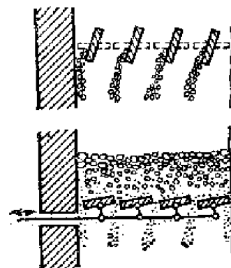
Рис. II.2. Схема действия поворотных и качающихся колосников
