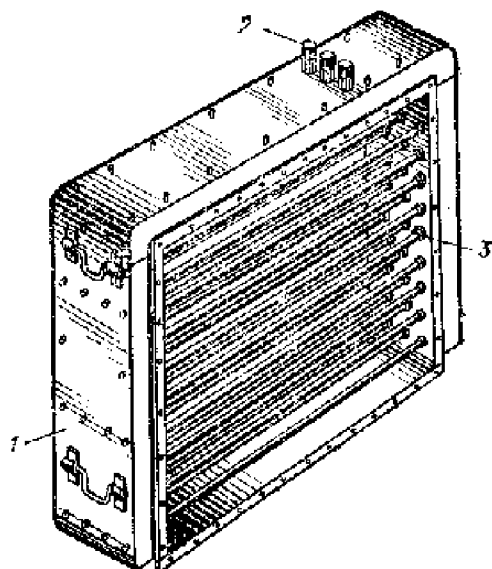
Рис. 111.26. Электрокалибратор 1 — корпус; 2 — подключение к электропроводке; 3 — нагревательные элементы.
