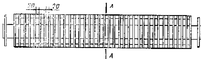
Рис. 11.58. Ребристая труба
