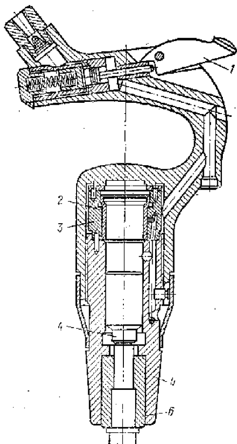
Рис. 1.27. Пневматический молоток
