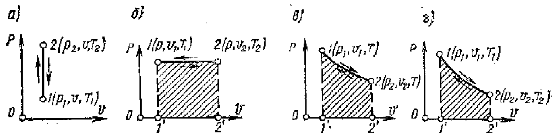
Рис. 1.6. Основные термодинамические процессы в координатах p-v
