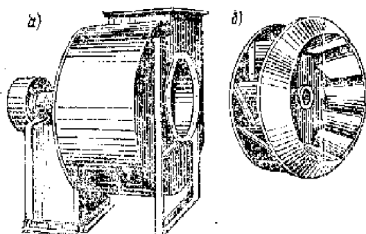
Рис. III.19. Центробежный вентилятор
