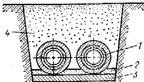
Рис. II.23. Бесканальная прокладка теплопроводов в монолитных оболочках из армированного пенобетона
