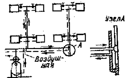
Рис. II.77. Система парового отопления с нижним распределением пара
