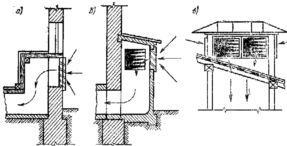
Рис. 11.30. Воздухоприсосные устройства
