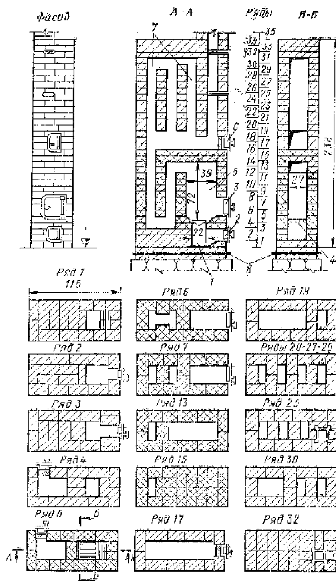
Рис. 11.89. Печь нижнего прогрева с теплоотдачей 3000 Bt
