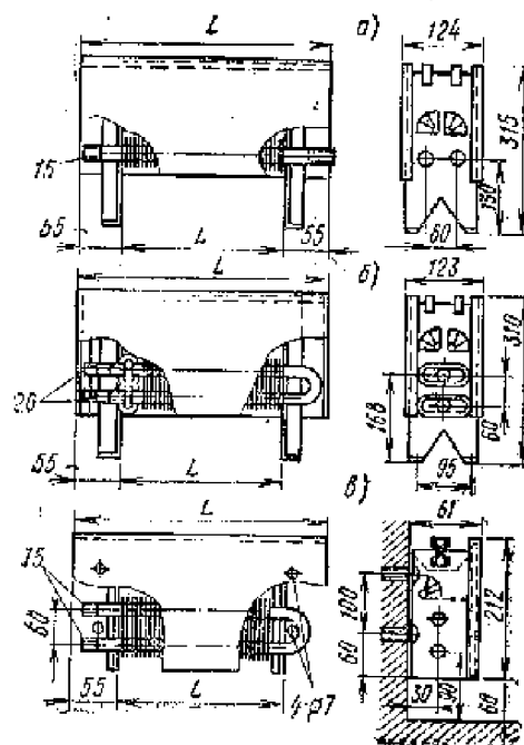
Рис. II.39. Конвектор «Аккорд»
