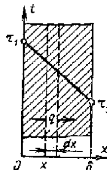
Рис. 1.29. Теплопроводность однослойной плоской стенки
