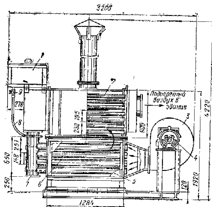
Рис. II.99. Воздухонагреватель
