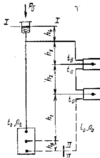
Рис. 11.57. Схема к определению естественного давления в проточной однотрубной системе водяного отопления
