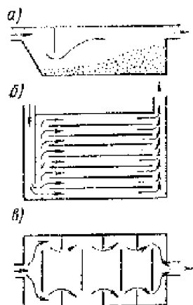
Рис. 11.38. Пылеосадочные камеры
