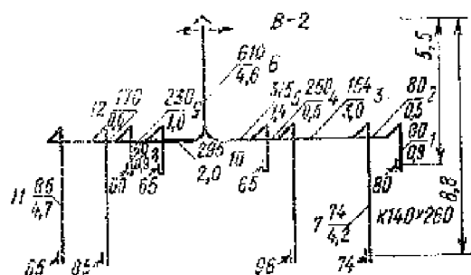
Рис. 11.11. Схема системы вытяжной вентиляции (к примеру расчета воздуховода)
