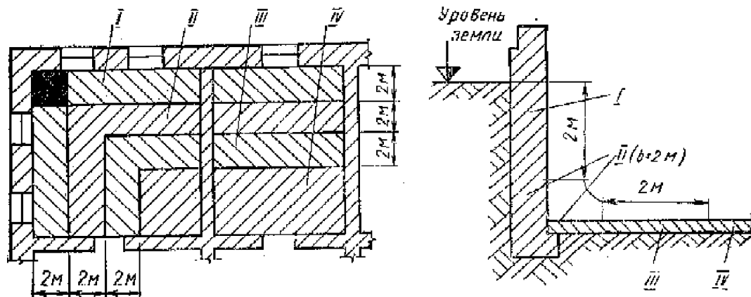
Рис. II.31. Схема к определению потерь тепла через полы и стены, заглубленные ниже уровня земли I — первая зона; II — вторая зона; III — третья зона; IV — четвертая зона (последняя)
