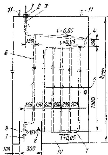
1 — металлическая пробка; 2 — муфта; 3 — участок стояка; 4 — верхний коллектор; 5 — трубы регистра; 6 — замыкающий участок; 7 — нижний коллектор; 8 — край двойной регулировки; 9 — тройник; 10 — отопительная панель; 11 — подвесные петли
