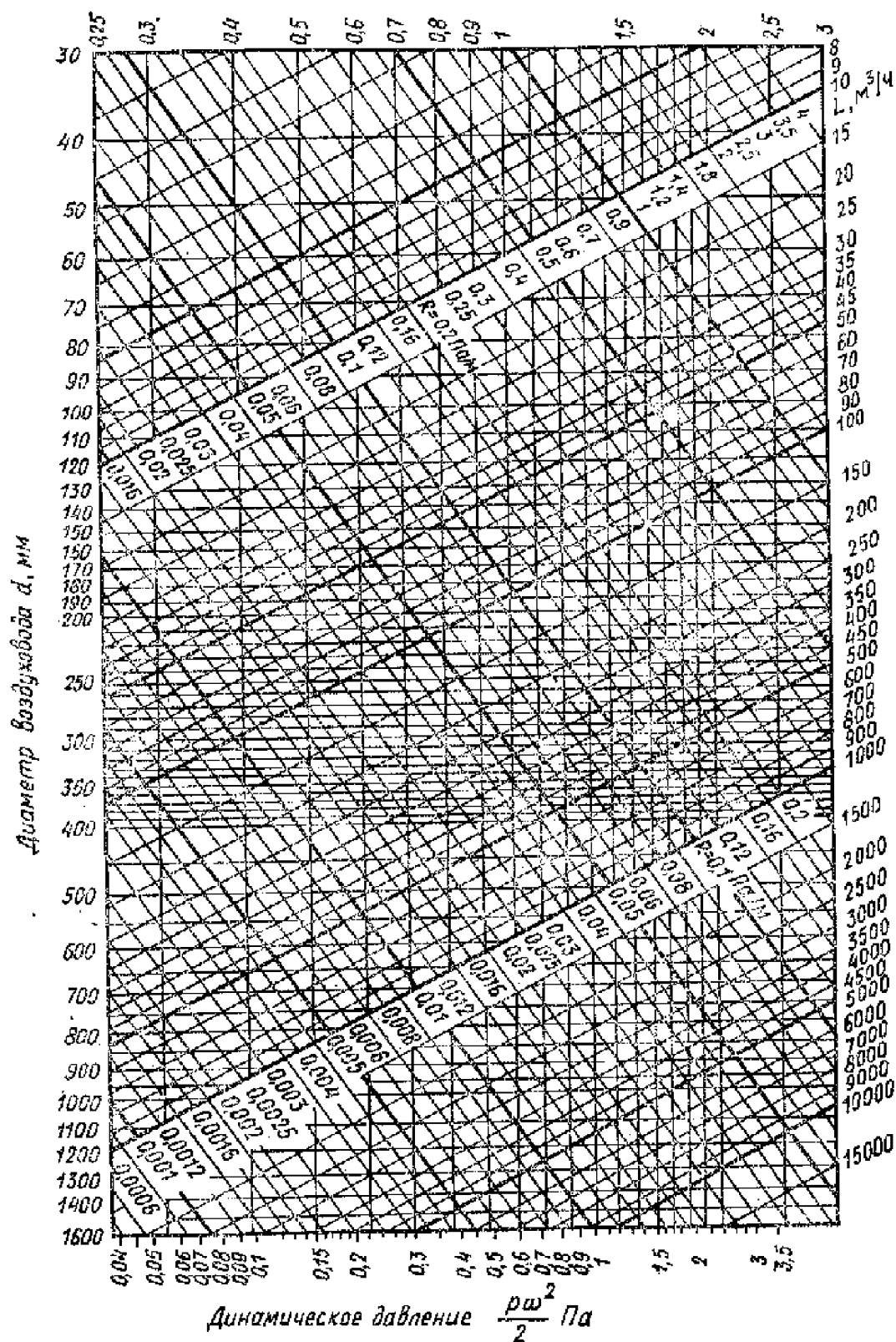
Рис. III.12. Номограмма для расчета круглых стальных воздуховодов
