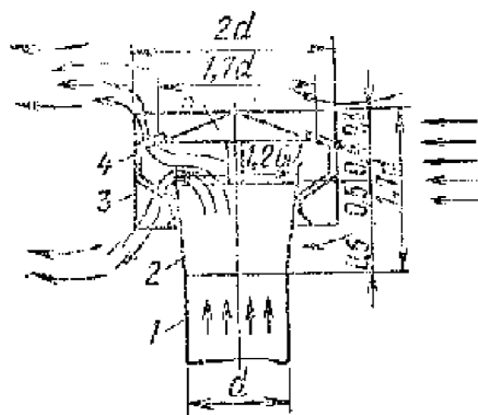
Рис. III.13. Дефлектор ЦАГИ
