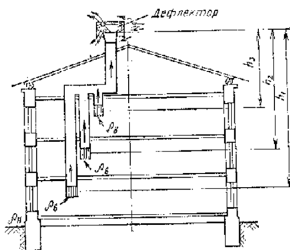
рис. 111.3. Схемы вытяжной естественной канальной вентиляции
