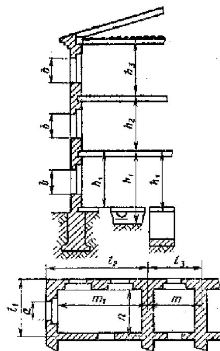
Рис. II.30. Правила обмера теплопередающих ограждений
