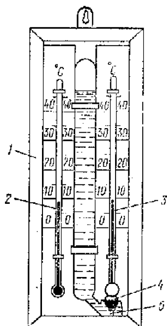
Рис. 1.16. Психрометр
