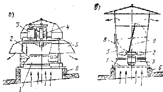
Рис. III.22. Крышные вентиляторы
