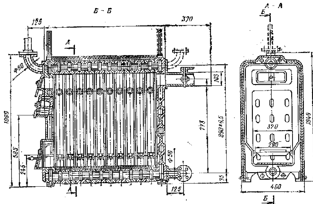
Рис. II.5. Чугунный водогрейный котел ВНИИСТО-мч
