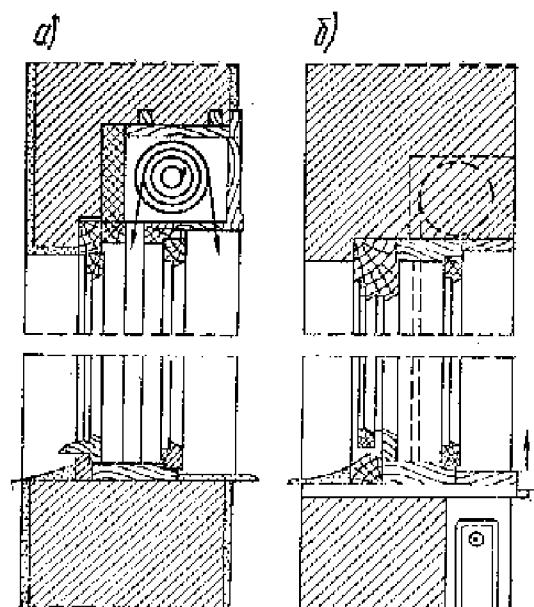
Рис. II.34. Окна с помещенной между рамами свертывающейся шторой а — с двойным остеклением; б — с тройным остеклением
