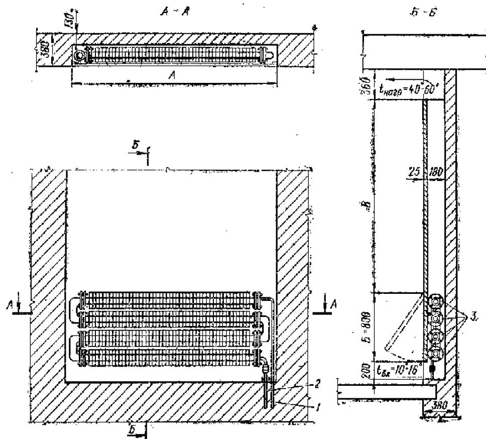
Рис. II.44. Рециркуляционный воздушнонагреватель для отопления лестничных клеток 1 — подающая труба; 2 — обратная труба; 3 — нагревательный элемент
