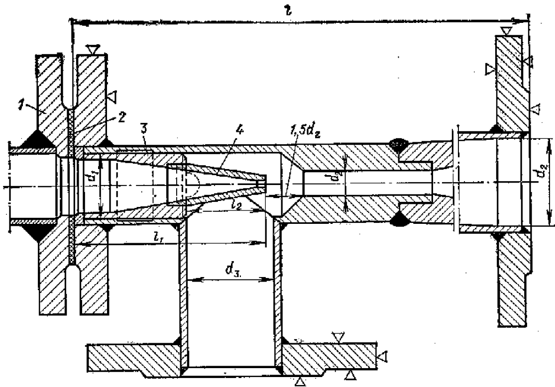
Рис. II.68. Элеватор
