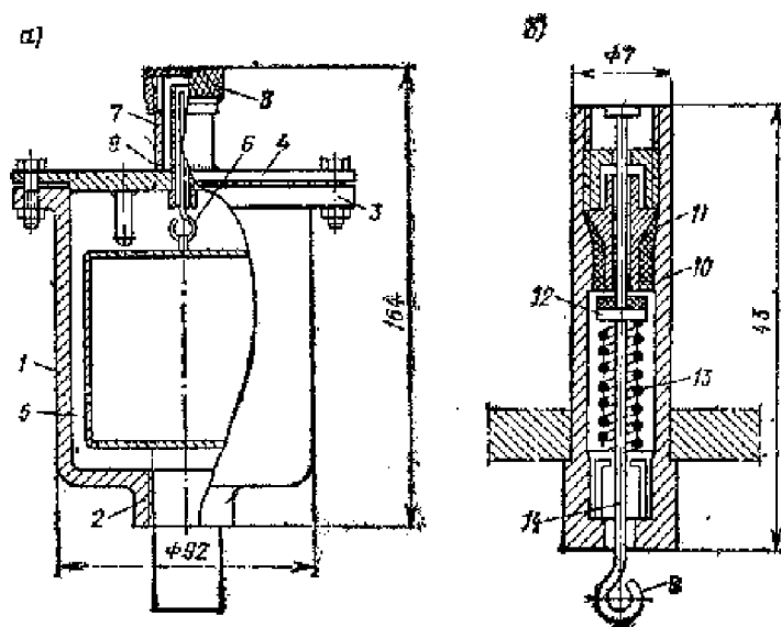
Рис. II.64. Автоматический воздухоотводчик ВНИИГС
