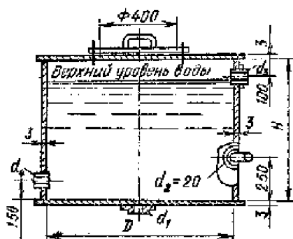
Рис. II.58. Расширительный сосуд
