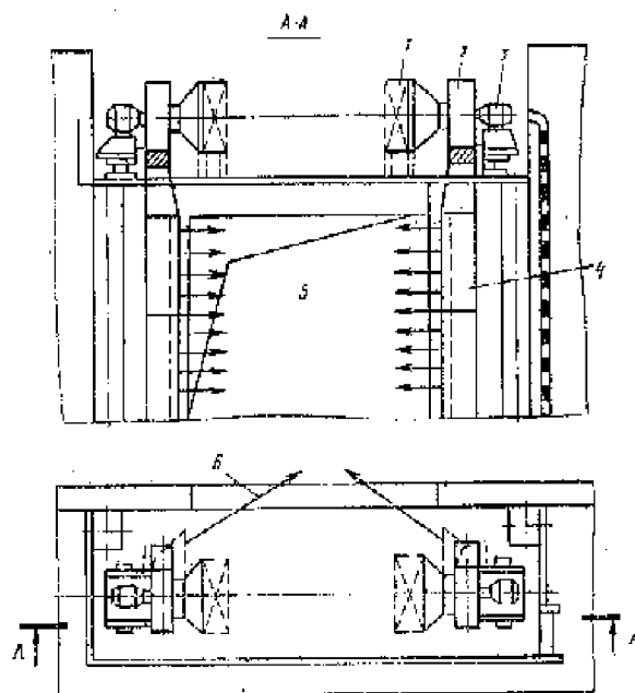
Рис. III.37. Воздушно-тепловая завеса
