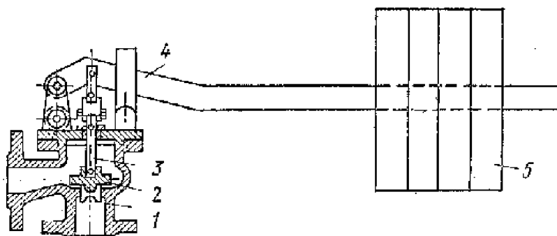
Рис. II.8. Предохранительный клапан
