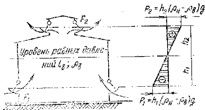
Рис. III.15. Схема аэрации зданий
