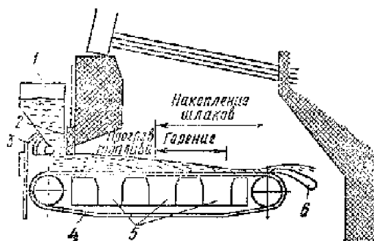
Рис. II.3. Топка с цепной решеткой 1 — бункер; 2 — шибер; 3 — затвор; 4 — движущаяся колосниковая решетка; 5 — подача воздуха; 6 — шлакоотсос
