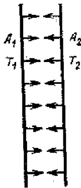
Рис. 1.32. Теплообмен излучением между двумя параллельными стенками
