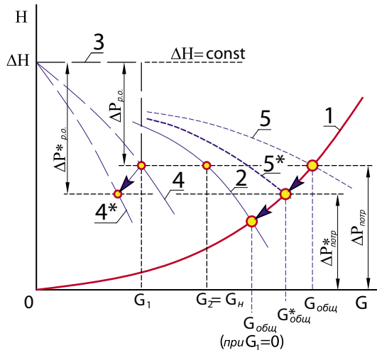
Рис.3.10.в. График характеристик сопротивлений в схеме узла смешения для второго варианта исходных условий
