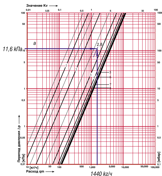
Рис. 4.5. Определение гидравлических характеристик вентиля балансировочного фланцевого ШТРЕМАКС-GMF, d25 с измерительными клапанами, арт.1421843 (поз.13а рис.4.1).
