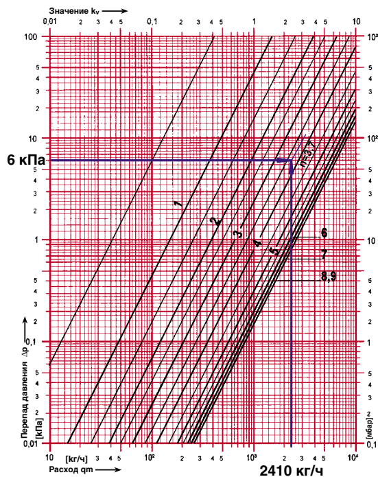
Рис. 4.53. Определение сопротивления вентиль балансового ШТРЕМАКС-GM, d40, арт.1421705 с измерительными клапанами, поз.3.2 рис.4.46.
