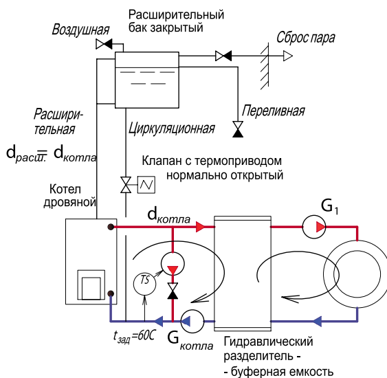
Рис. 4.42. Общая схема двухконтурной системы теплотребления с буферной емкостью в качестве гидравлического разделителя
