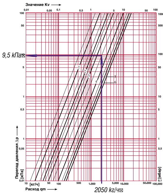
Рис. 4.13. Определение сопротивления вентиля балансирового фланцевого ШТРЕМАКС-GMF, d32 с измерительными клапанами, арт.1421844 (поз.4 рис.4.13).
