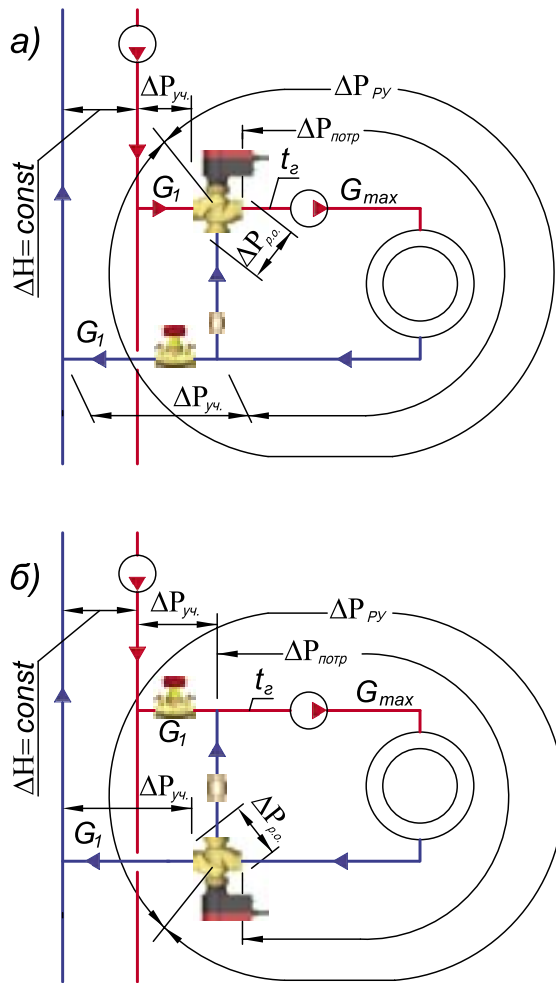
Рис. 3.15. Расчетная первая схема узла смешения со смесительным насосом на магистральном теплопроводе системы теплоснабжения
