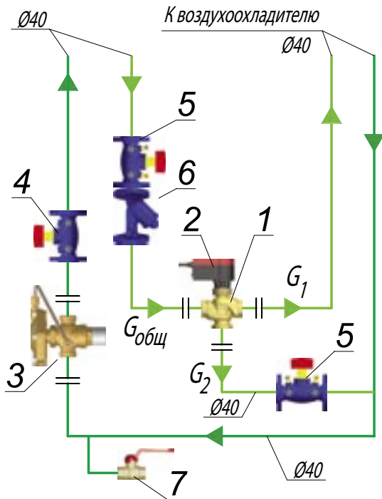
Рис. 4.23. Узел регулирования воздухоохладителей кондиционеров П2 и П3 1 – клапан ГЕРЦ арт.14037; 2 – электропривод ГЕРЦ арт.1771211; 3 – регулятор расхода арт.1400126; 4 – вентиль запорный фланцевый ШТРЕМАКС-AGF, арт.4218 AGF; 5 – вентиль балансировочный фланцевый ШТРЕМАКС-GMF с измерительными клапанами, арт.4218 GMF; 6 – фильтр-грязевик ГЕРЦ, арт.14111; 7 – кран дренажный.
