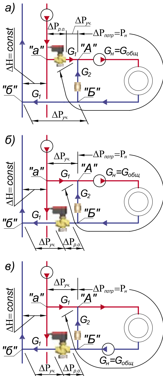
Рис.3.11. Расчетная первая схема узла смешения со смесительным насосом на магистральном теплопроводе системы теплоснабжения
