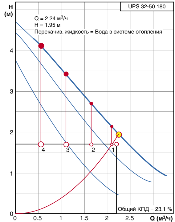
Рис. 4.57. Расчетная характеристика циркуляционного насоса UPS 32-50 180 (поз.Р4.1 рис.4.46)
