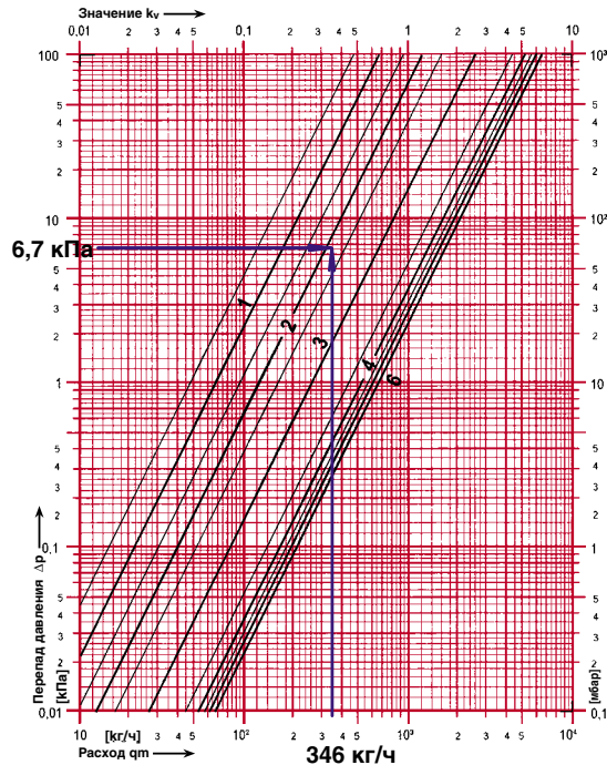
Рис. 4.87. Определение гидравлической преднастройки балансового вентиля ШТРЕМАКС-GM, d20, арт.1421702 поз.12 фэнкойла №10 для создания сопротивления 6,7кПа при расходе воды 346кг/ч.
