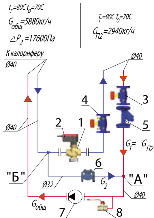
Рис. 4.15. Узел регулирования «2»
