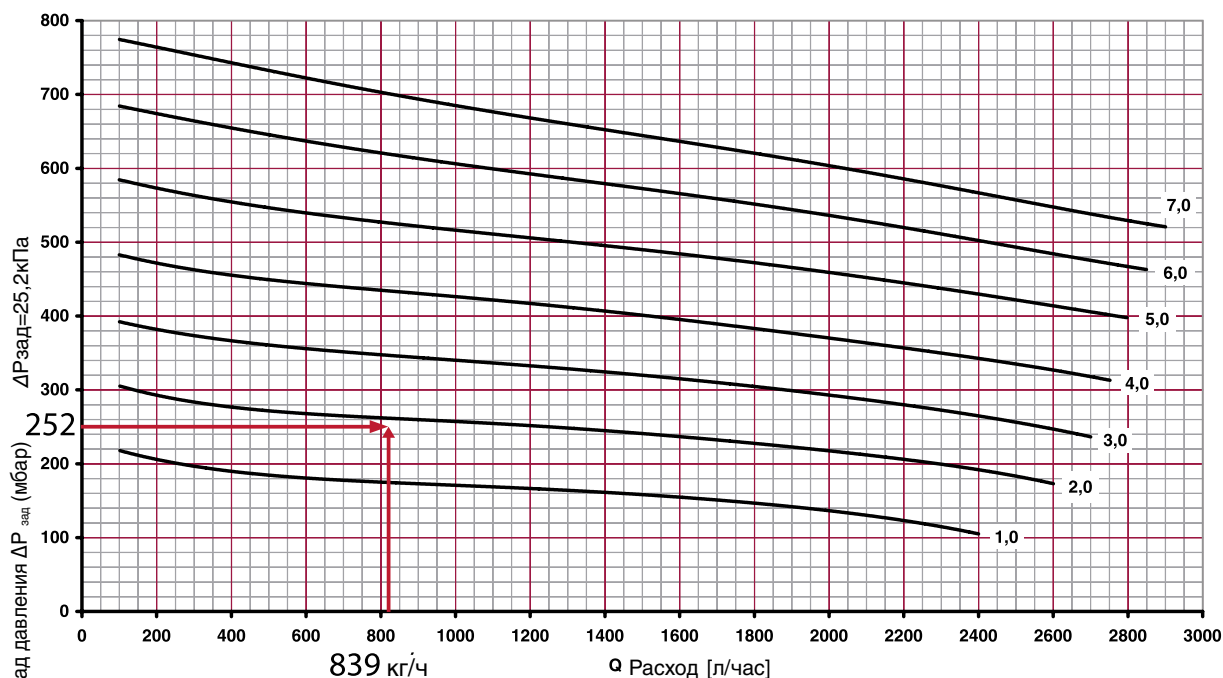
Рис. 4.73. Определение значения гидравлической настройки (n=1,9) регулятора перепада давления ГЕРЦ 4002, d25, арт.1400243 (поз.8 рис.4.59 ветки «В») при задаваемых расчетных значениях G_{порт}=839\text{кг/ч} и \Delta P_{зад}=25,2\text{кПа}
