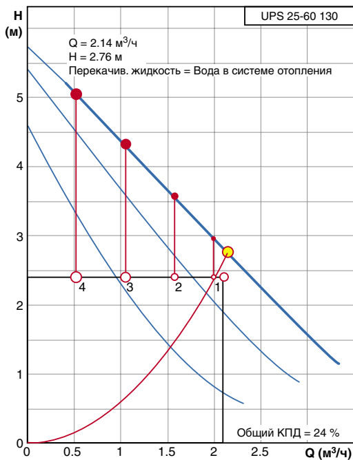
Рис.4.52. Расчетная характеристика смесительного насоса UPS 25-60 130 (поз.Р2.1 рис.4.46)
