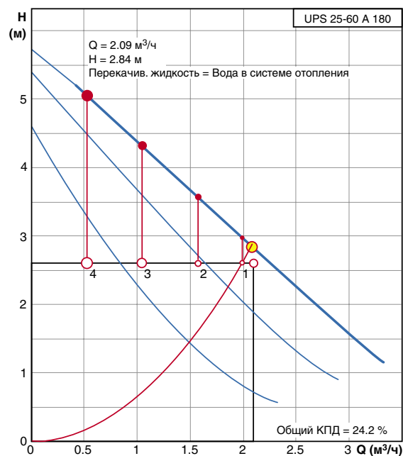
Рис.4.35. Расчетная характеристика смесительного насоса UPS 25-60 A 180 (поз.Р2.1 рис.4.28)
