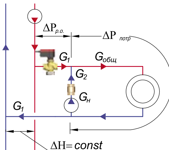
Рис. 3.10.а. Расчетная схема узла смешения со смесительным насосом на перемычке
