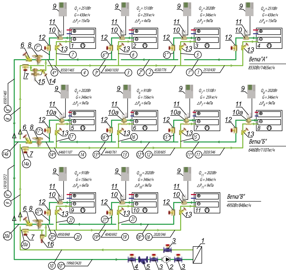
Рис. 4.74. Схема расчетная системы холодоснабжения четырехтрубных фэнкойлов
