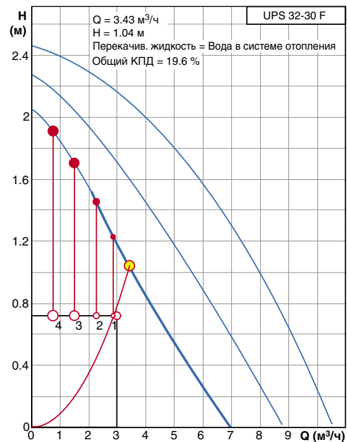
Рис. 4.48. Расчетная характеристика циркуляционного насоса UPS 32-30 F (поз. P1.2 рис.4.46)
