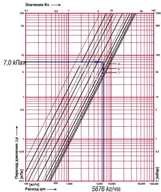
Рис. 4.92. Определение значения гидравлической преднастройки вентиля балансировочного фланцевого ШТРЕМАКС-GMF, d50 с измерительными клапанами, арт.1421846 (поз.4 рис.4.91) при расчетных значениях \Delta P_{\text{в.4}}=7,0 кПа и G_{\text{в.4}}=5676 кг/ч.
