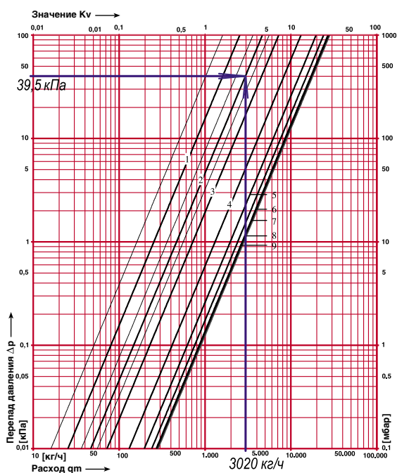
Рис 4.24. Определение значения гидравлической преднастройки вентиля балансового фланцевого ШТРЕМАКС-GMF, d40 с измерительными клапанами, арт.1421845 (поз.5 рис.4.23) при расчетных значениях \Delta P_{в.5}=39,5 кПа и G_{в.5}=3020 кг/ч.
