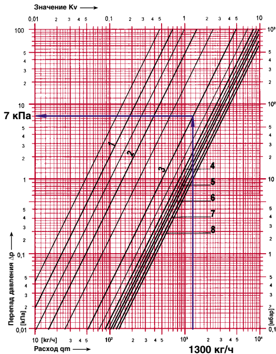
Рис. 4.39. Определение сопротивления вентилей балансового ШТРЕМАКС-GM, d25, арт.1421703 с измерительными клапанами, поз.4.2 рис.4.28.
