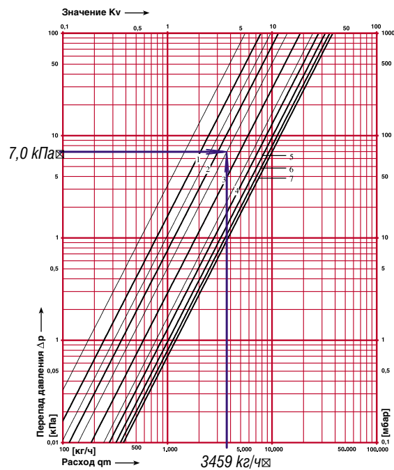
Рис. 4.61. Определение значения гидравлической преднастройки вентиля балансировочного фланцевого ШТРЕМАКС-GMF, d50 с измерительными клапанами, арт.1421846 (поз.4 рис.4.59) при расчетных значениях \Delta P_{в.4} = 7,0\text{кПа} и G_{в.4} = 3459\text{кг/ч} .
