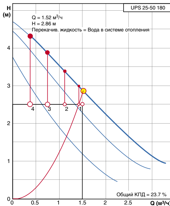
Рис. 4.49. Расчетная характеристика смесительного насоса UPS 25-50 180 (поз.Р1.2 рис. 4.46)
