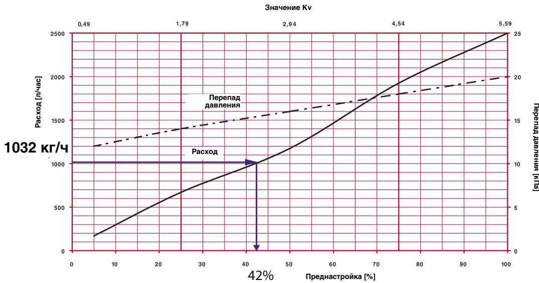
Рис. 4.93. Определение значения гидравлической настройки регулятора расхода ГЕРЦ 4001, d32, арт.1400124 (поз.8 рис.4.91 на системе отопления аудитории №6) при расчетном значении G_{общ} = 1032 \text{ кг/ч} .
