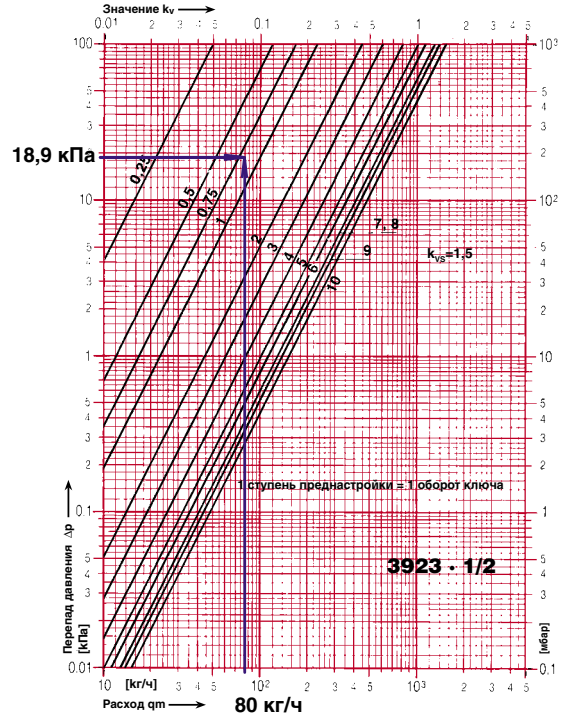
Рис.4.102. Определение значения гидравлической преднастройки вентиля балансового ГЕРЦ RL-5, арт.1392301, d15 (поз.3.1 рис.4.97) при значениях P_{б.в.3.1}=18,9\text{кПа} и G_{б.в.3.1}=80\text{кг/ч} .
