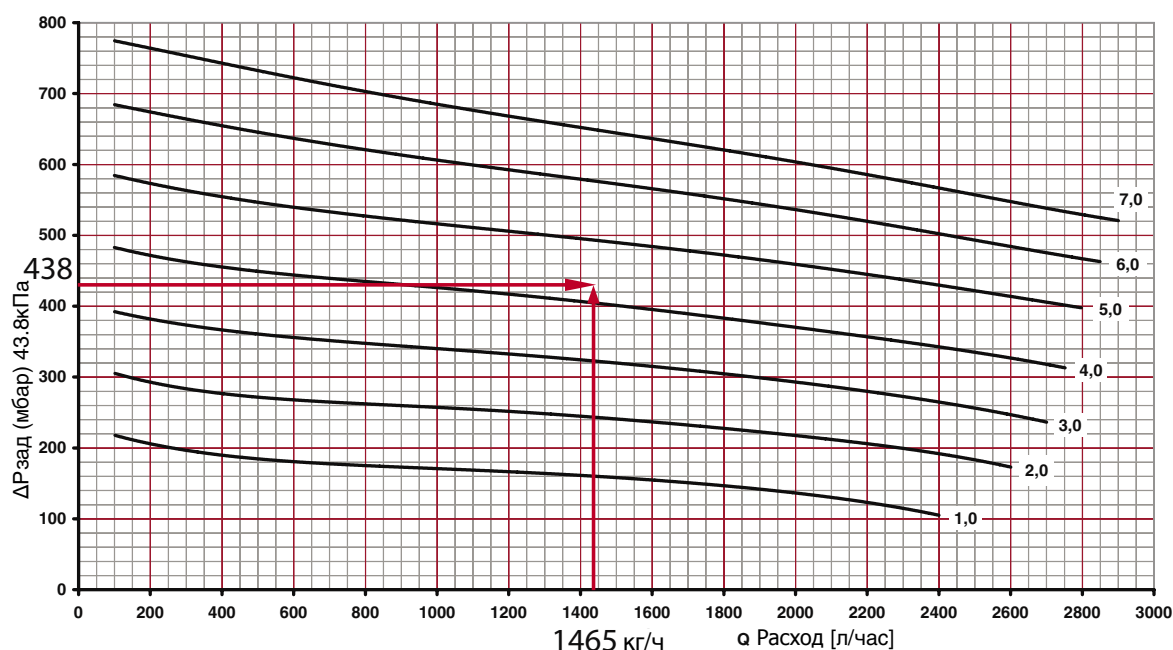
Рис.4.81. Определение значения гидравлической настройки ( n=4,6 ) регулятора перепада давления ГЕРЦ 4002, d25, арт.1400263 (поз.15 рис.4.74 ветки «А») при задаваемых расчетных значениях G_{потр} = 1465 \text{ кг/ч} и \Delta P_{зад} = 43.8 \text{ кПа}
