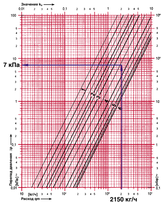
Рис. 4.56. Определение сопротивления вентиля балансировочного ШТРЕМАКС-GM, d32, арт.1421704 с измерительными клапанами, поз.4.2 рис.4.46.
