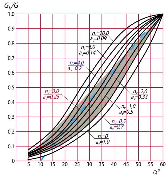
Рис. 3.6. Расходные характеристики поворотной заслонки.
