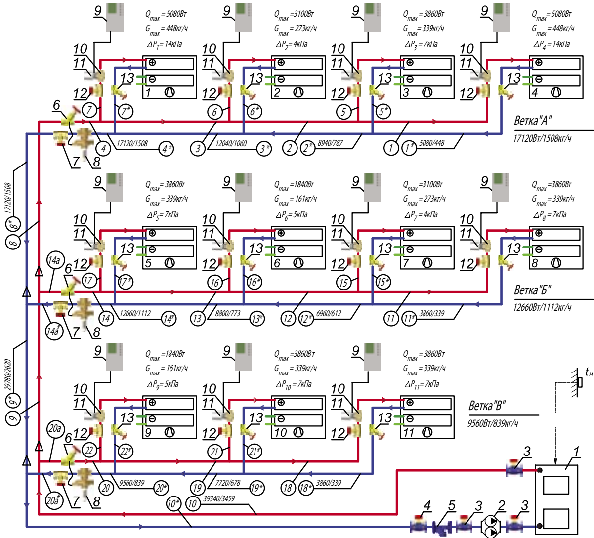
Рис. 4.59. Схема расчетная системы теплоснабжения четырехтрубных фэнкойлов 1 – котел 45кВт на природном газе; 2 – насос циркуляционный; 3 – вентиль запорный фланцевый ШТРЕМАКС-AGF, арт.4218 AGF; 4 – вентиль балансировочный фланцевый ШТРЕМАКС-GMF с измерительными клапанами, арт.4218 GMF; 5 – фильтр-грязевик ГЕРЦ 4111; 6 – вентиль запорный ШТРЕМАКС-A арт.14115; 7 – вентиль балансировочный ШТРЕМАКС-GM арт.14217; 8 – регулятор перепада давления ГЕРЦ 4002; 9 – регулятор электронный непрерывного действия арт.7794; 10 – двухходовой термостатический клапан арт.17760 0X; 11 – термопривод арт. 7711 NO; 12 – вентиль балансировочный ШТРЕМАКС-GM арт.14217; 13 – вентиль запорный ШТРЕМАКС-A арт.14115.
