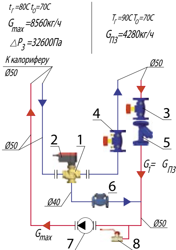
Рис. 4.19. Узел регулирования «3»
