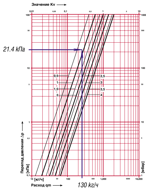
Рис.4.103. Определение значения гидравлической преднастройки вентиля балансового ШТРЕМАКС 4017М арт.1401711, d15 (поз.4.1 рис.4.97) при расчетных значениях \Delta P_{б.б.4.1} = 21,4 \text{ кПа} и G_{б.б.4.1} = 130 \text{ кг/ч} .
