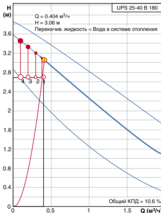
Рис.4.100. Расчетная характеристика циркуляционного насоса UPS 25-40 В 180 (поз.Р2 рис.4.97)
