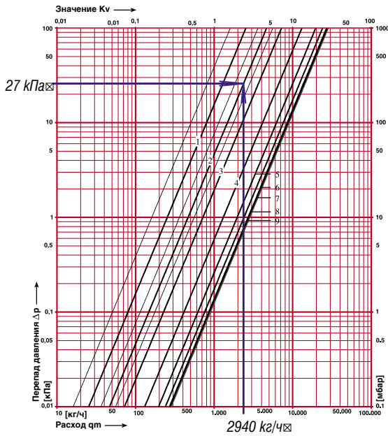
Рис. 4.17. Определение значения гидравлической преднастройки вентиля балансового фланцевого ШТРЕМАКС-GMF, d40 с измерительными клапанами, арт.1421845 (поз.4 рис.4.15) при расчетных значениях \Delta P_{\beta,4} = 27\text{кПа} и G_{\beta,4} = 2940\text{кг/ч} .
