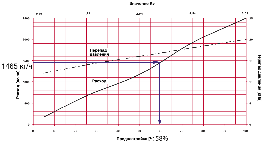
Рис. 4.82. Определение значения гидравлической настройки регулятора расхода ГЕРЦ 4001, d32, арт.1400124 (поз.8 ветки «А» рис.4.74 при расчетном значении G_{общ}=1465\text{кг/ч} .
