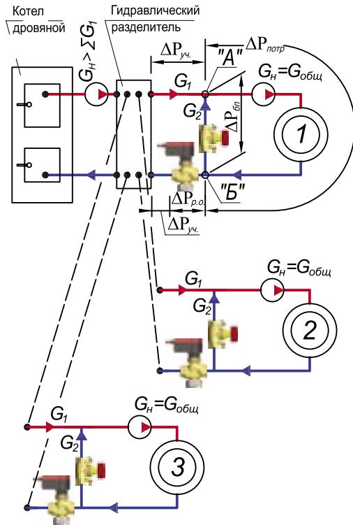
Рис.3.13. Расчетная вторая схема для узлов смешения со смесительным насосом на магистральном теплотрассе системы теплоснабжения (при параллельном присоединении систем теплоснабжения к гидравлическому разделителю)
