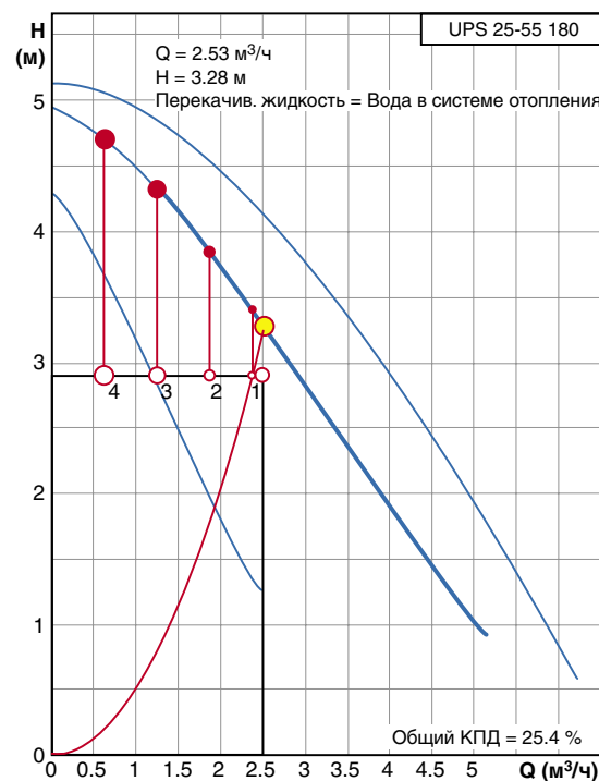
Рис. 4.55. Расчетная характеристика смесительного насоса UPS 25-55 180 (поз.РЗ.1 рис.4.46)
