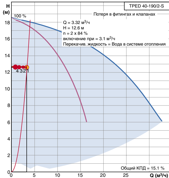
Рис. 4.67. Расчетная характеристика циркуляционного насоса TPED 40-190/2-S (поз.2 рис.4.59)
