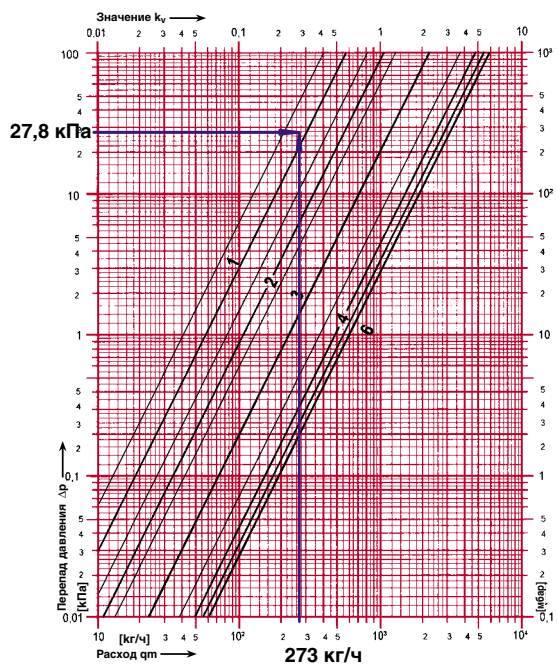
Рис.4.64. Определение гидравлической преднастройки балансового вентиля ШТРЕМАКС-GM, d15, арт.1421701 поз.12 фэнкойла №2 для создания сопротивления 27,8кПа при расходе теплоносителя 273кг/ч.
