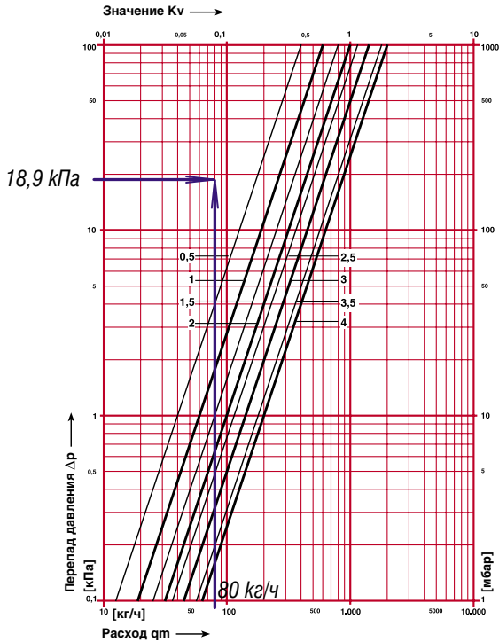
Рис.4.101. Определение значения гидравлической преднастройки вентиля балансового ШТРЕМАКС 4017М арт.1401711, d15 с измерительными клапанами, (поз.3.1 рис.4.97) при значениях \Delta P_{б.в.3.1}=18,9\text{кПа} и G_{б.в.3.1}=80\text{кг/ч} .
