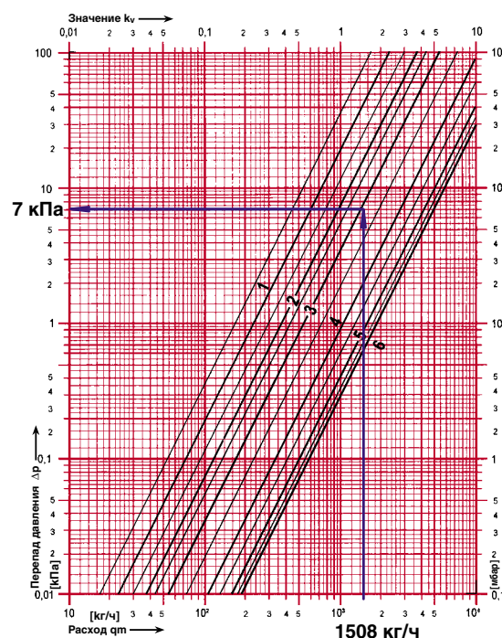
Рис. 4.60. Определение сопротивления вентиля балансового ШТРЕМАКС-ГМ, d32, арт.1421704 с измерительными клапанами, поз.7 рис.4.59.
