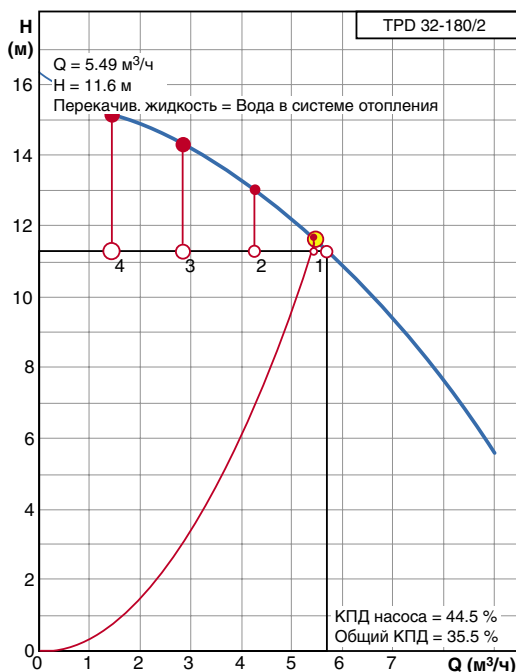
Рис. 4.94. Расчетная характеристика циркуляционного насоса Grundfos TPD 32-180/2 (поз.2 рис.4.91)
