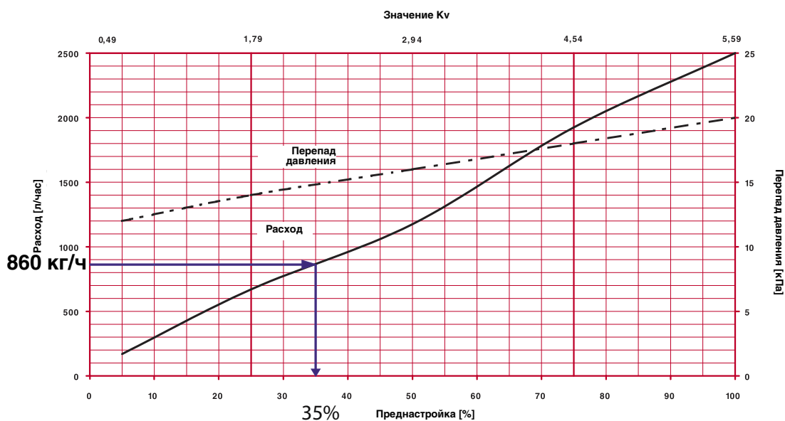
Рис.4.96. Определение значения гидравлической настройки регулятора расхода ГЕРЦ 4001, D32, арт.1400123 (поз.8 рис.4.91 на системе отопления аудитории №5) при расчетном значении G_{общ} = 860 \text{ кг/ч} .
