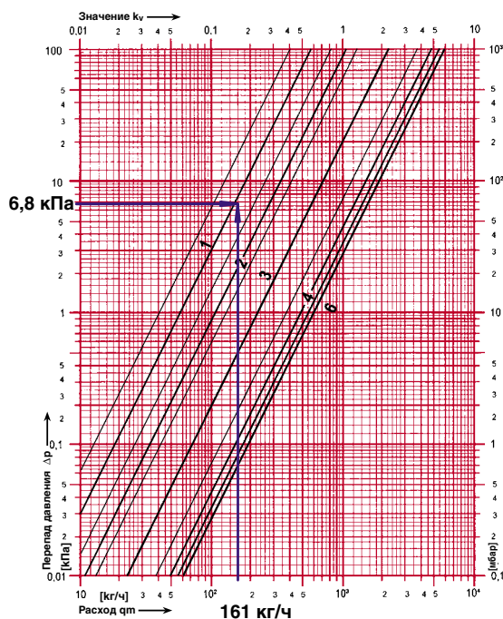
Рис. 4.72. Определение гидравлической преднастройки балансировочного вентиля ШТРЕМАКС-ГМ, d15, арт.1421701 поз.12 фэнкойла №9 для создания сопротивления 6,8кПа при расходе теплоносителя 161кг/ч.
