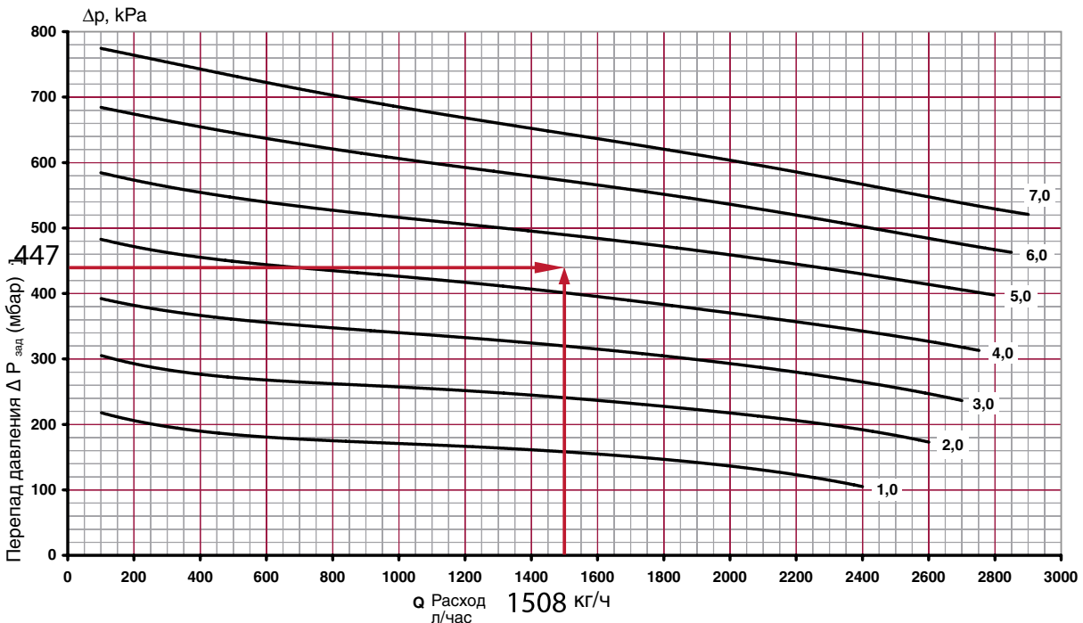
Рис. 4.66. Определение значения гидравлической настройки ( n=4.7 ) регулятора перепада давления ГЕРЦ 4002, d25, арт.1400263 (поз.8 рис.4.59 ветки «А») при задаваемых расчетных значениях G_{\text{потр}}=1508 кг/ч и \Delta P_{\text{заг}}=44.7 кПа
