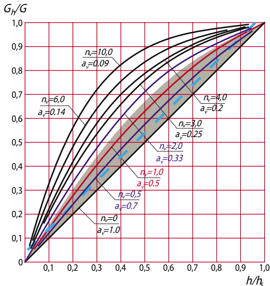
Рис. 3.4. Расходные характеристики РО с линейной пропускной характеристикой.
