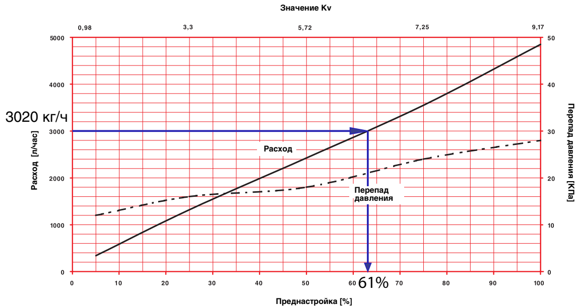
Рис. 4.25. Определение значения гидравлической настройки регулятора расхода ГЕРЦ 4001, d50, арт.1400126 (поз.3 рис. 4.23 для воздухоохладителя установки П2 при расчетном значении G_{общ} = 3020 \text{ кг/ч} .)
