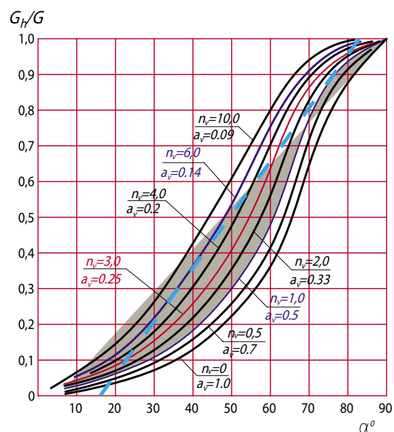
Рис. 3.7. Расходные характеристики запорно-регулирующей заслонки ГЕРЦ 4219
