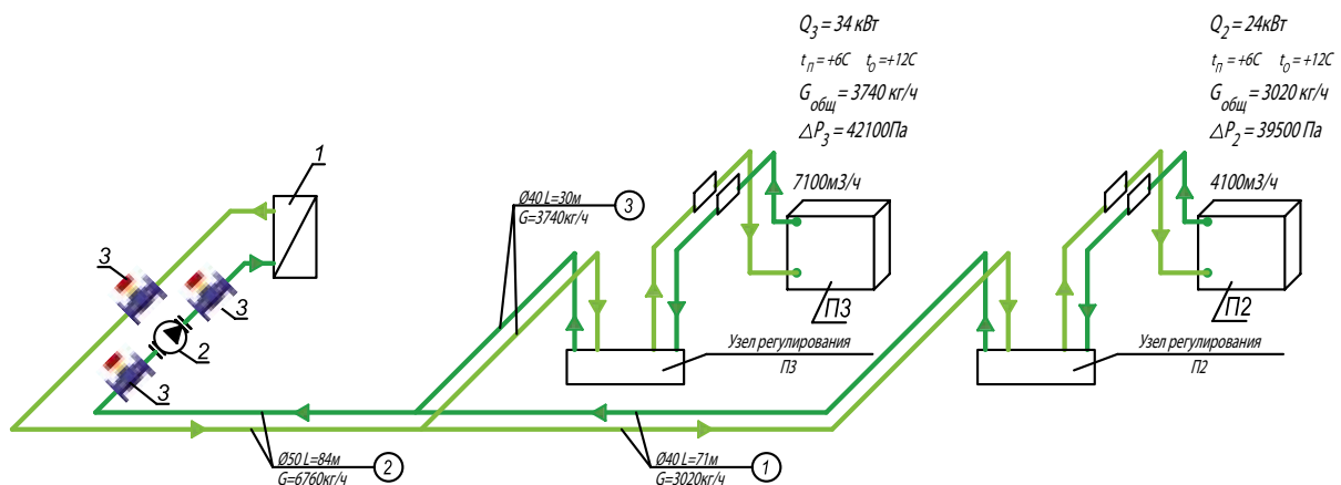
Рис. 4.22. Схема системы холодоснабжения воздухоохлаждающих кондиционеров П2 и ПЗ с исходными данными для гидравлического расчета и подбора оборудования 1 – испаритель чиллера; 2 – насос циркуляционный водяной; 3 – вентиль запорный фланцевый ШТРЕМАКС-AGF, арт.4218 AGF.
