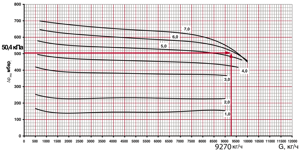
Рис. 4.14. Определение значения гидравлической настройки регулятора перепада давления ГЕРЦ 4002, d50, арт.1400266 (поз. 3 рис. 4.11) для системы теплоснабжения калориферов при задаваемых расчетных значениях G_{номр} = 9270 \text{ кг/ч} и \Delta P_{заг} = 50,4 \text{ кПа} .
