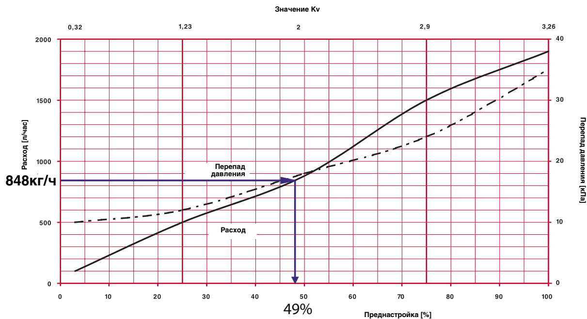
Рис. 4.90. Определение значения гидравлической настройки регулятора расхода ГЕРЦ 4001, d25, арт.1400123 (поз.8 ветки «В» рис.4.74 при расчетном значении G_{\text{общ}}=848\text{кг/ч} ).
