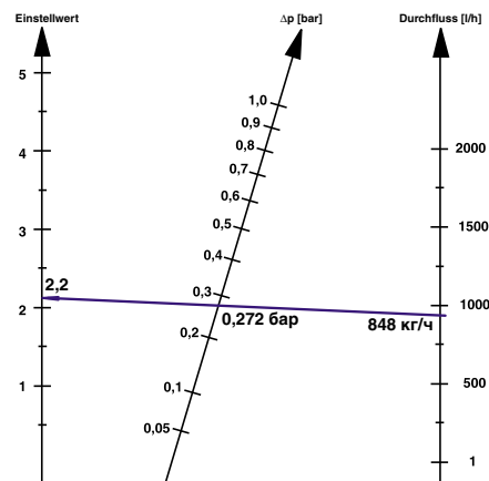
Рис.4.89. Определение значения гидравлической настройки ( n=2,2 ) перепускного клапана ГЕРЦ 4004, d20, арт.1400442 (поз.16 рис.4.74 ветки «В») при задаваемых расчетных значениях G_{\text{номп}}=848 \text{ кг/ч} и \Delta P_{\text{заг}}=0,272 \text{ бар} .
