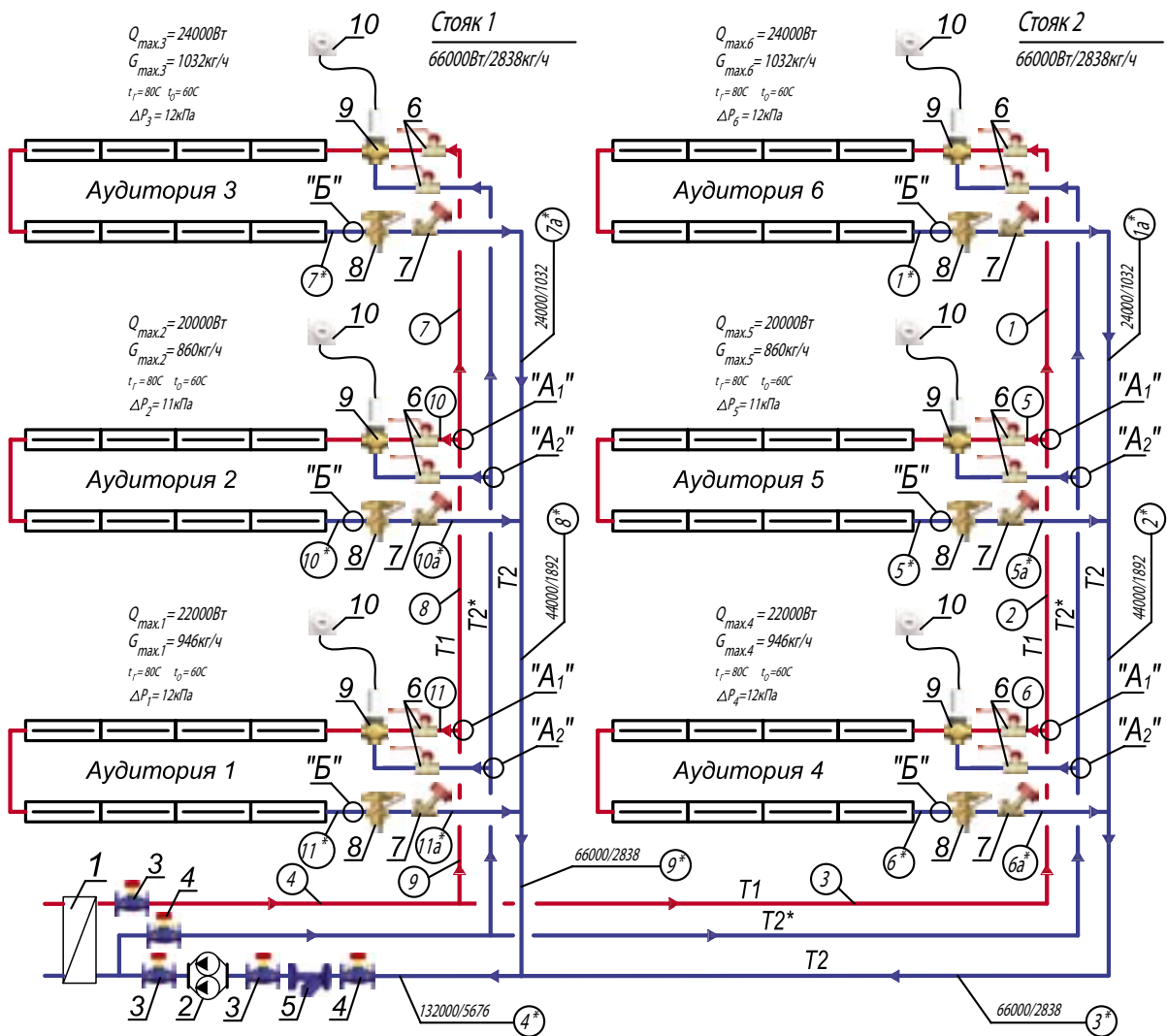
Рис. 4.91. Схема расчетная трехтрубной системы отопления поточных учебных аудиторий
