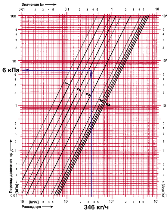
Рис. 4.86. Определение сопротивления вентиля балансового ШТРЕМАКС-GM, d20, арт.1421702 с измерительными клапанами, поз.12 рис.4.74, для фэнкойла №11.
