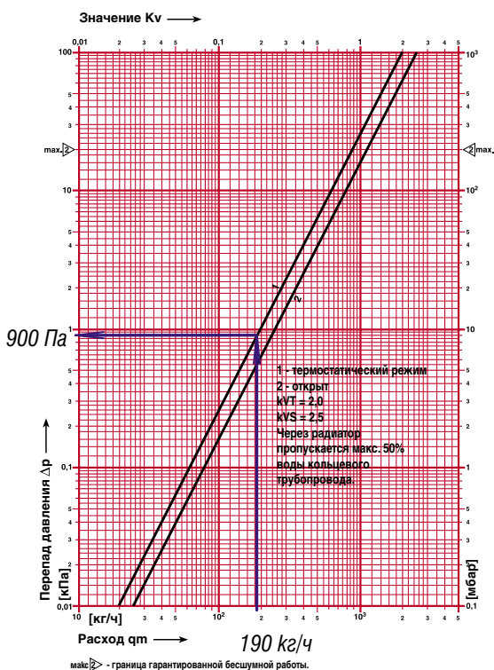
Рис. 4.99. Определение \Delta P_{\text{кв1}} узла подключения ГЕРЦ-2000 (поз.2.5 рис.4.97)
