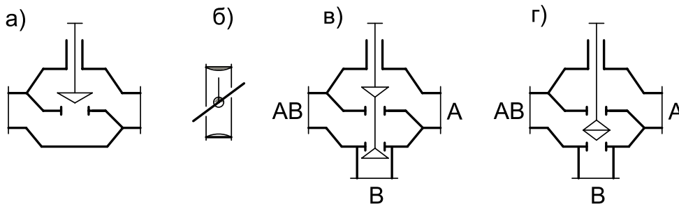
Рис. 3.2. Типы регулирующих органов а) двухходовой (проходной) седельный регулирующий орган; б) заслонка поворотная; в), г) трехходовой регулирующий орган.
