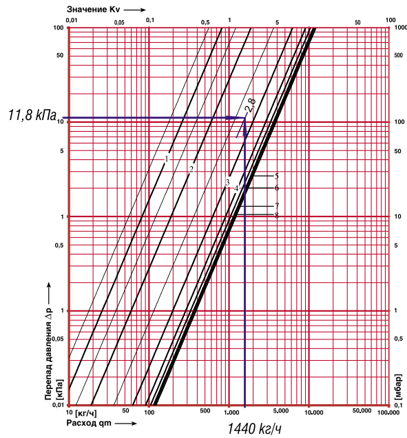
Рис. 4.9. Определение гидравлических характеристик вентиля балансирового фланцевого ШТРЕМАКС-GMF, d25 с измерительными клапанами, арт.1421843 (поз.13а рис.4.7).
