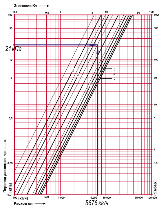
Рис.4.95. Определение значения гидравлической преднастройки вентиля балансового фланцевого ШТРЕМАКС-GMF, d50 с измерительными клапанами, арт.1421846 (поз.4 на теплопроводе Т2* рис.4.91) при расчетных значениях \Delta P_{в.4^*}=21,0\text{кПа} и G_{в.4^*}=5676\text{кг/ч} .
