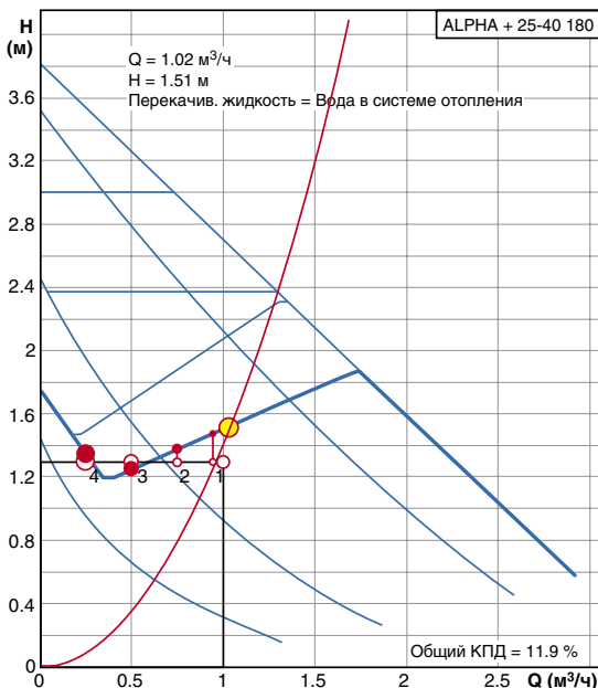
Рис. 4.29. Расчетная характеристика подмешивающего насоса ALPHA +25-40 180 (поз.4 рис. 4.28)
