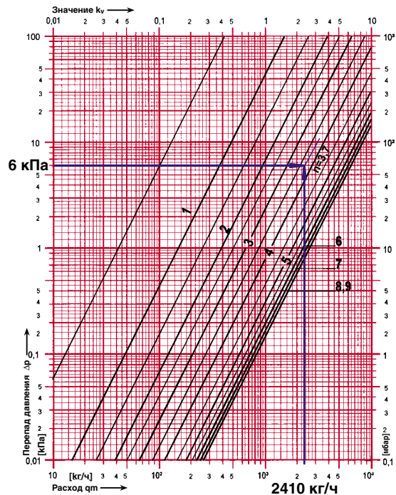
Рис. 4.36. Определение сопротивления вентиля балансового ШТРЕМАКС-GM, d40 , арт.1421705 с измерительными клапанами, поз. 3.2 рис. 4.28.
