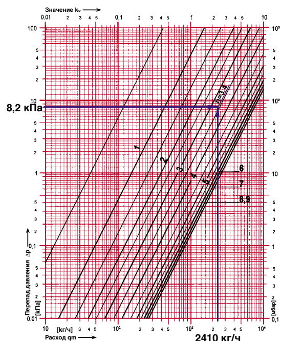
Рис. 4.54. Определение значения гидравлической преднастройки вентиль балансового ШТРЕМАКС-GM, d40, арт.1421705 с измерительными клапанами, поз.3.1 рис.4.46.
