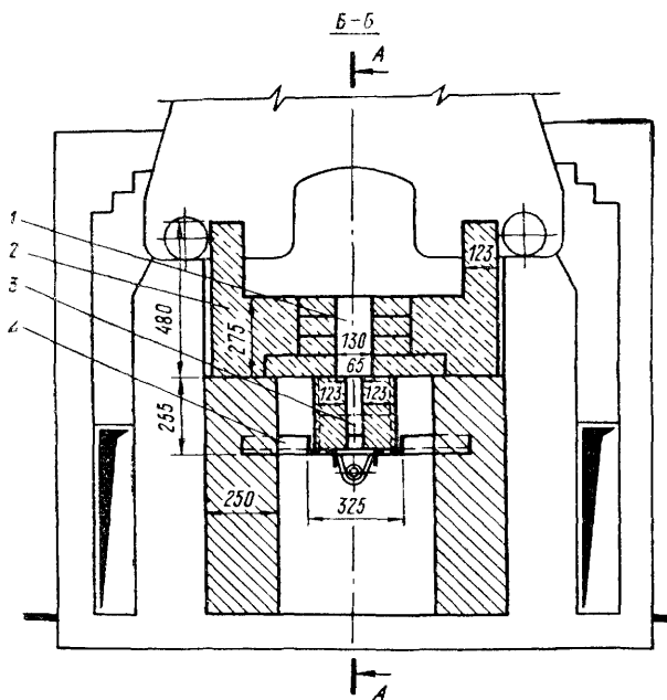
Рис. XII.9. Установка форкамерной горелки среднего давления на котлах «Универсал-6» и «Энергия-6» (по Укргипроинжпроект).
