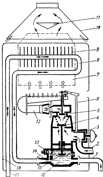
Рис. XI.4. Принципиальная схема газового водонагревателя ВПГ-18.
