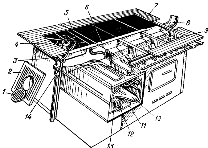
Рис. XI.11. Плита типа ПГР-1М.
