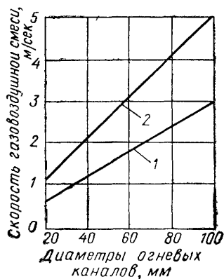
Рис. X.5. Максимальные скорости проскака пламени (в пересчете на 0° С и 760 мм рт. ст.) инжекционных однофакельных горелок для смесей природных газов с воздухом при \alpha = 1,0 :
