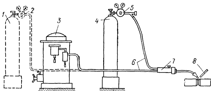
Рис. VII.3. Схема поста газовой сварки.
