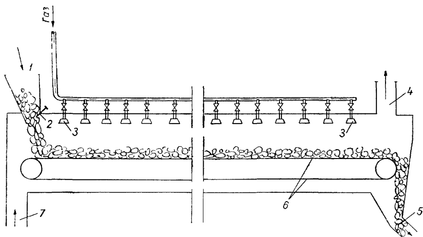
Рис. XIII.12. Принципиальная схема туннельной сушилки.
