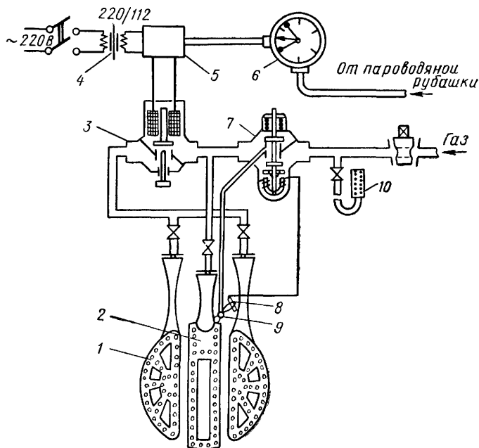
Рис. XI.14. Схема автоматики безопасности и регулирования котла КИП-250.
