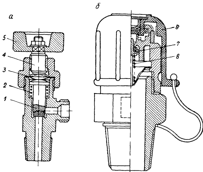
Рис. XIV.5. Вентили баллонные ВБ-1 (а) и самозакрывающийся КБ-1 (б).
