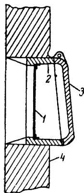
Рис. XII.4. Предохранительный взрывной клапан.
