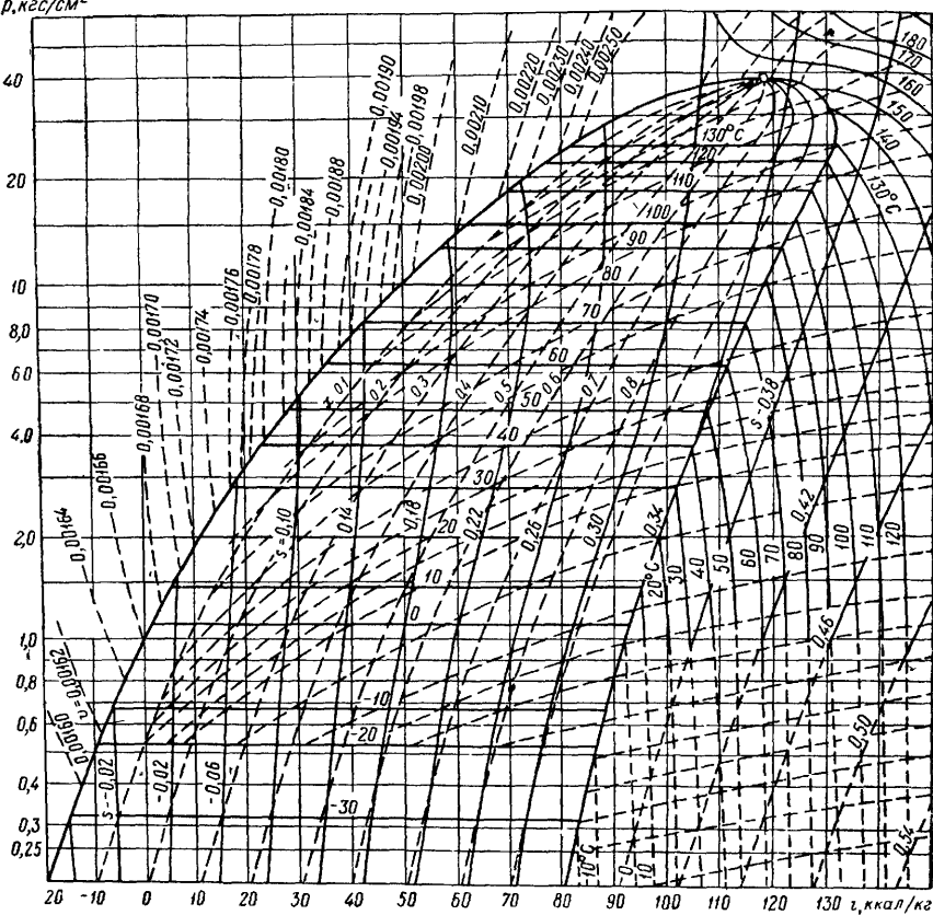
Рис. 11.3. Диаграмма состояния n -бутана.
