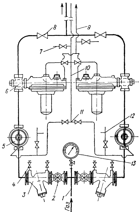
Рис. V.17. Принципиальная схема шкафового ГРП типа ШП-2 (ШП-3).
