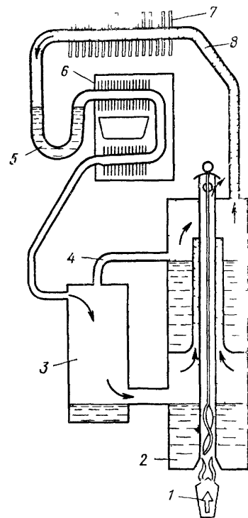
Рис. XI.9. Схема холодильного аппарата.
