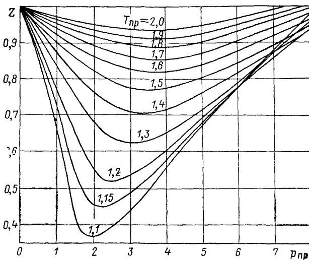
Рис. II.1. Коэффициенты сжимаемости газов Z в зависимости от приведенных температуры T_{пр} и давления p_{пр} при p_{пр} \leq 8,0 .
