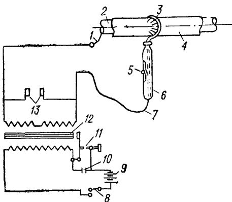
Рис. VIII.8. Схема искрового дефектоскопа Ленгаза.
