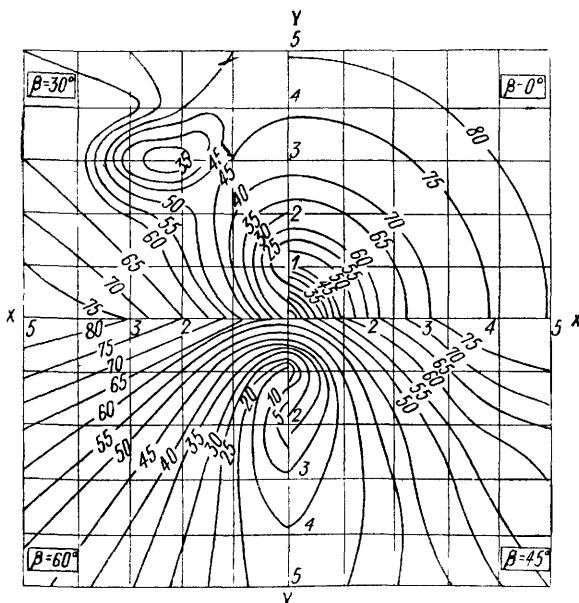
Рис. XIII.7. Номограмма для определения пространственного угла \alpha .
