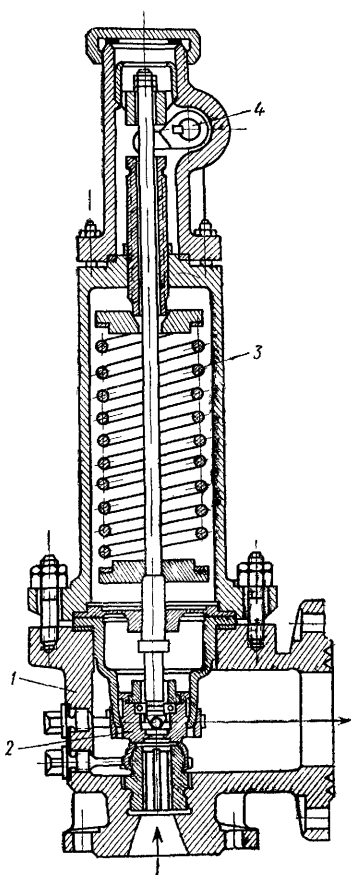
Рис. V.8. Предохранительный пружинный клапан ППК-4 (ППК-4ДМ).
