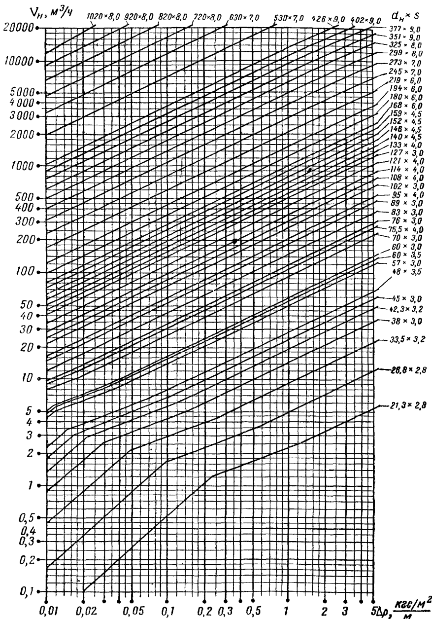
Рис. VI.3. Номограмма для определения удельных потерь давления в газо- проводах низкого давления (природный газ, \rho = 0,73 \text{ кг/м}^3 , \nu = 14,3 \times \times 10^{-6} \text{ м}^2/\text{сек} ).
