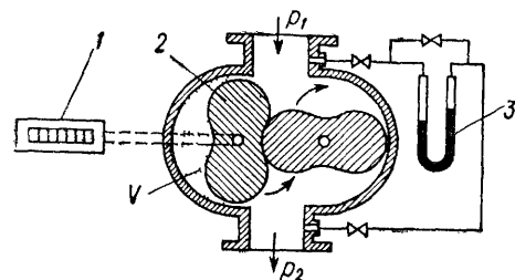
Рис. V.14. Схема ротационного счетчика.
