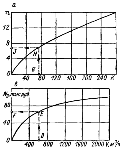
Рис. XIII.1. Графики для определения числа ГРП в сельских населенных пунктах.
