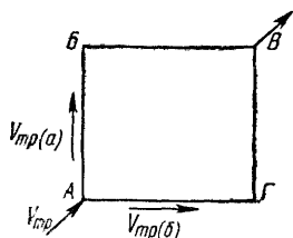
Рис. IV.2. Элемент кольцевой сети.
