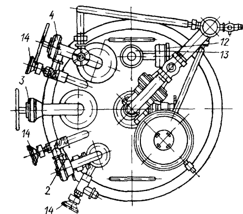
Рис. XIV.12. Головка подземного резервуара.
