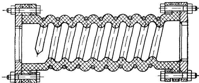
Рис. IV.9. Резинотканевый компенсатор.
