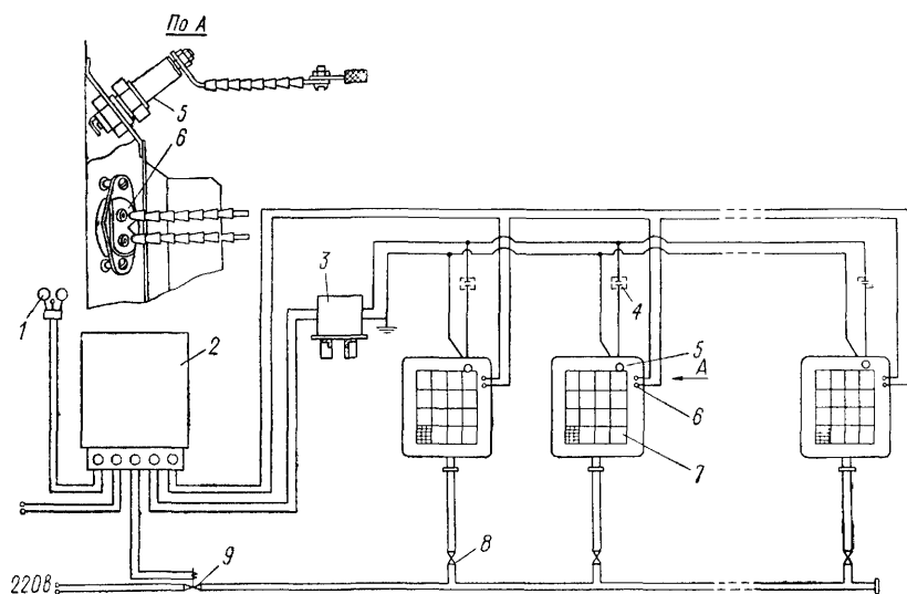
Рис. XIII.9. Схема автоматики зажигания и контроля горения горелок инфракрасного излучения «Искра».
