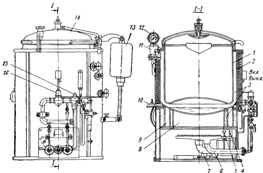
Рис. XI.13. Котел пищеварочный типа КПР-250.
