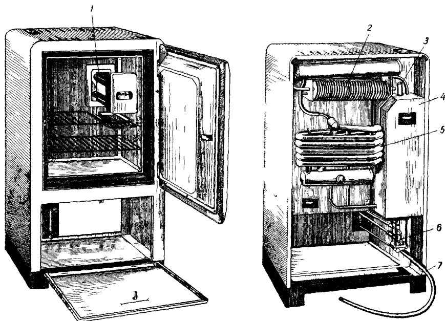
Рис. ХІ.8. Холодильник «Север-2».
